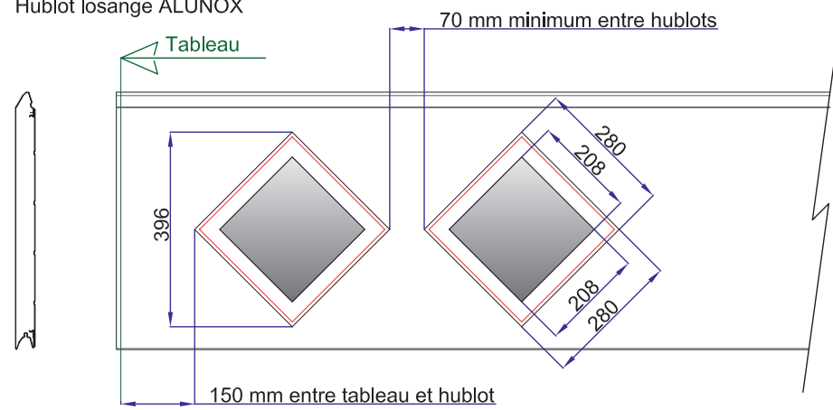
Hublot losange ALUNOX
