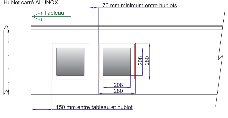
Hublot carré ALUNOX
